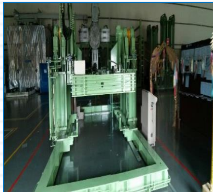
Machine de Levée des Bobines
